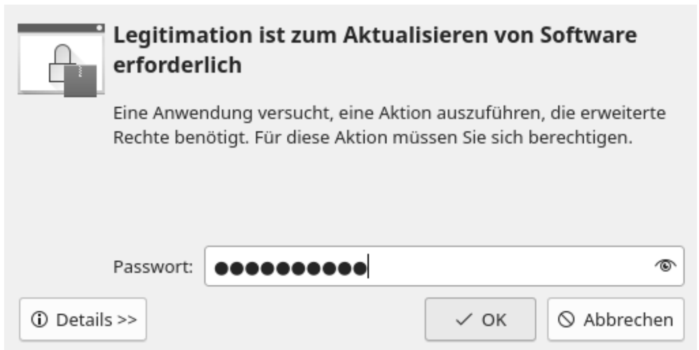
Discover: Passwortabfrage für die Aktualisierung
