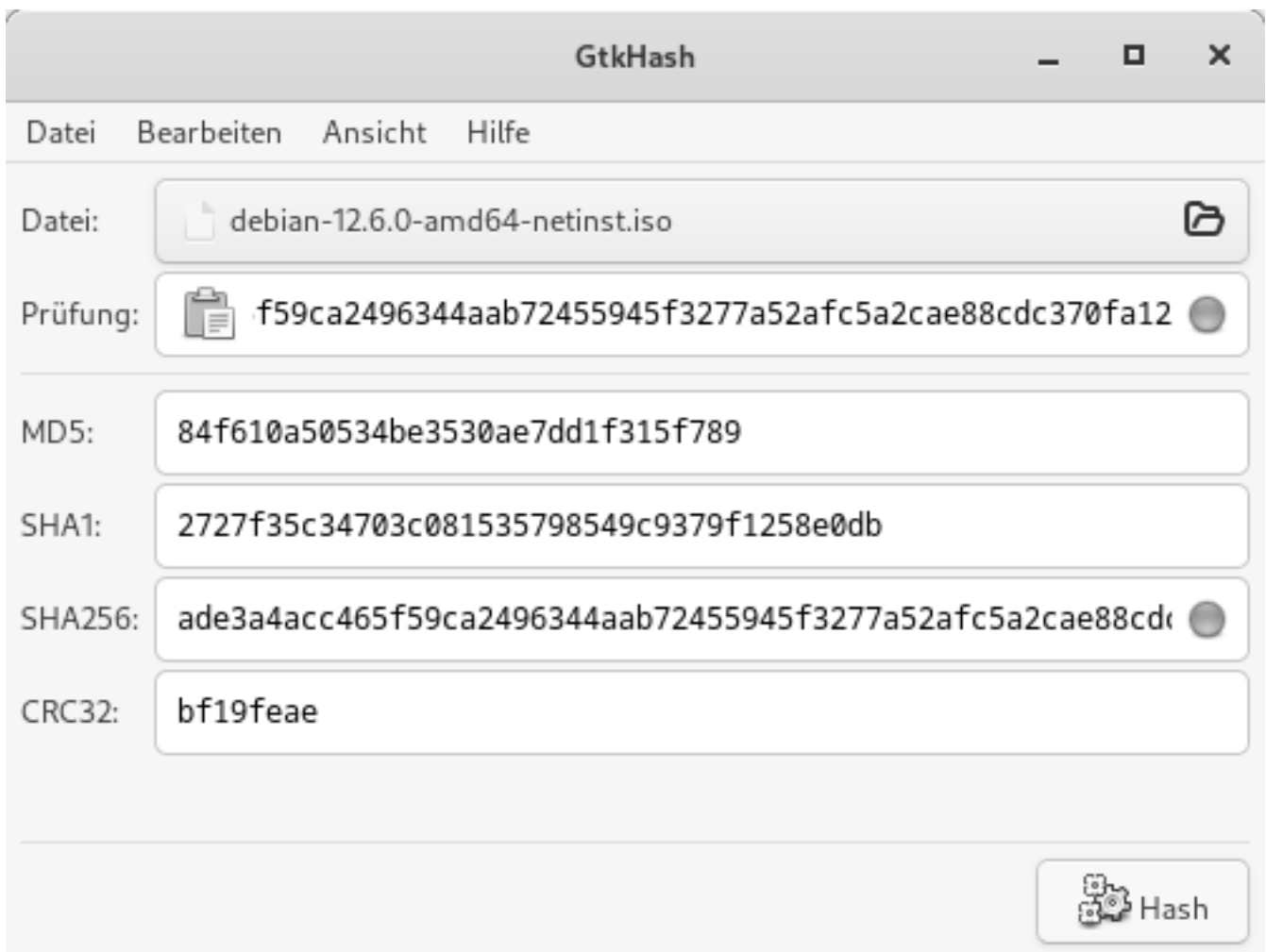
GtkHash: Überprüfung der SA256 Prüfsumme
