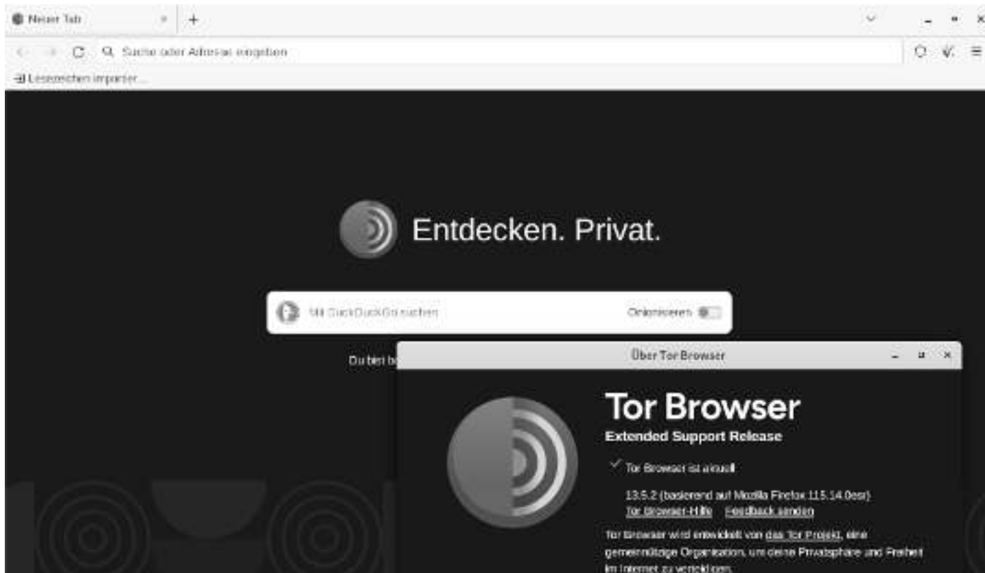
Tor Browser
