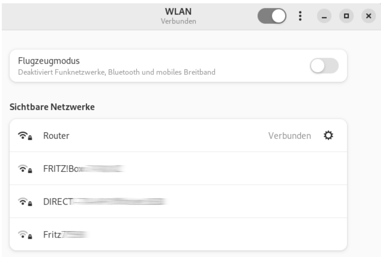
Netzwerkauswahl
