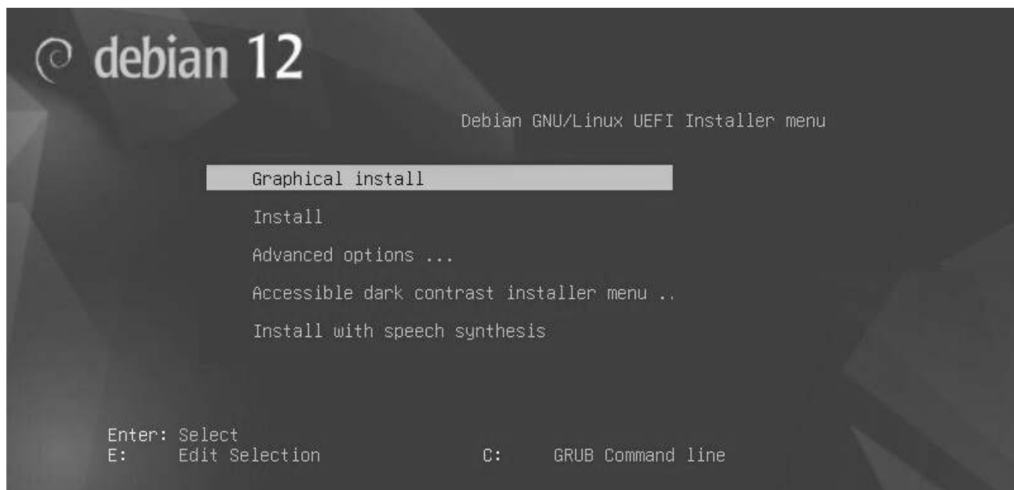
Installationsmodus (UEFI)
