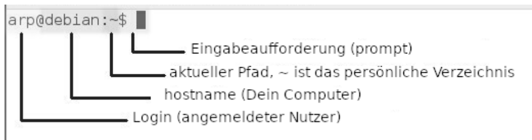
Terminal Präsentation
