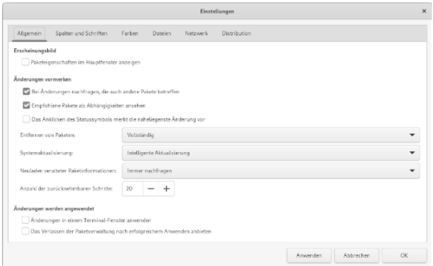
Synaptic: Einstellungsfenster
