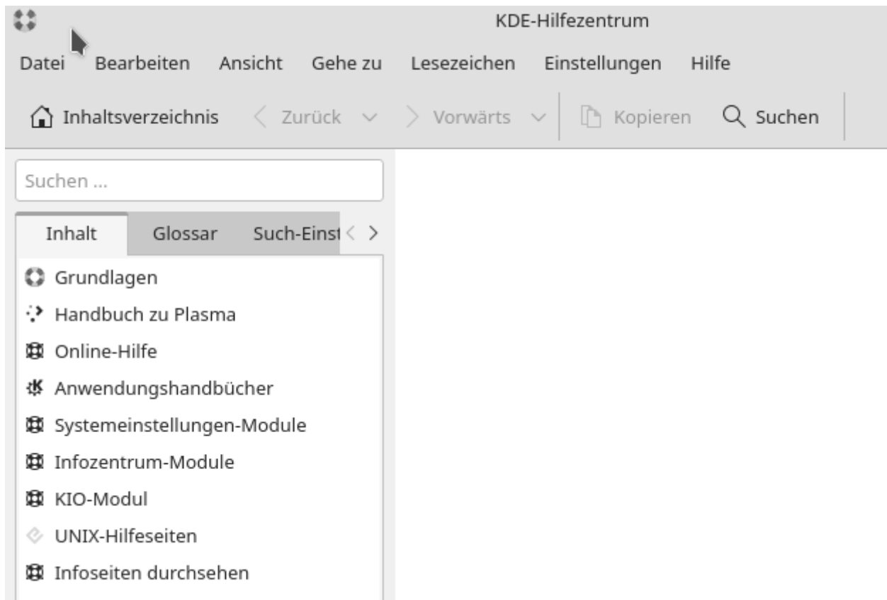
KDE Hilfezentrum
