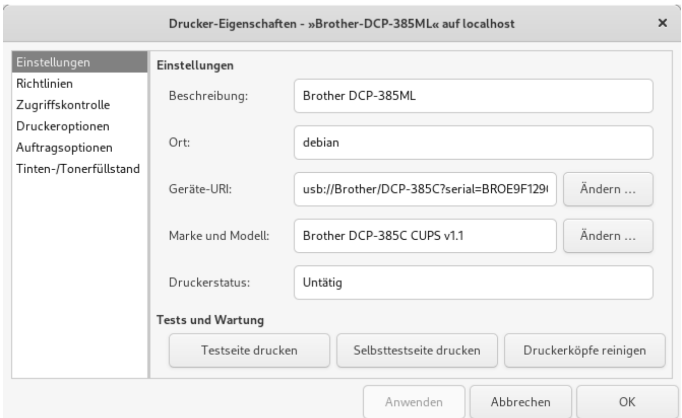
Druckereinstellungen
