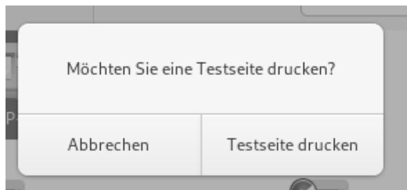
Testseite drucken?
