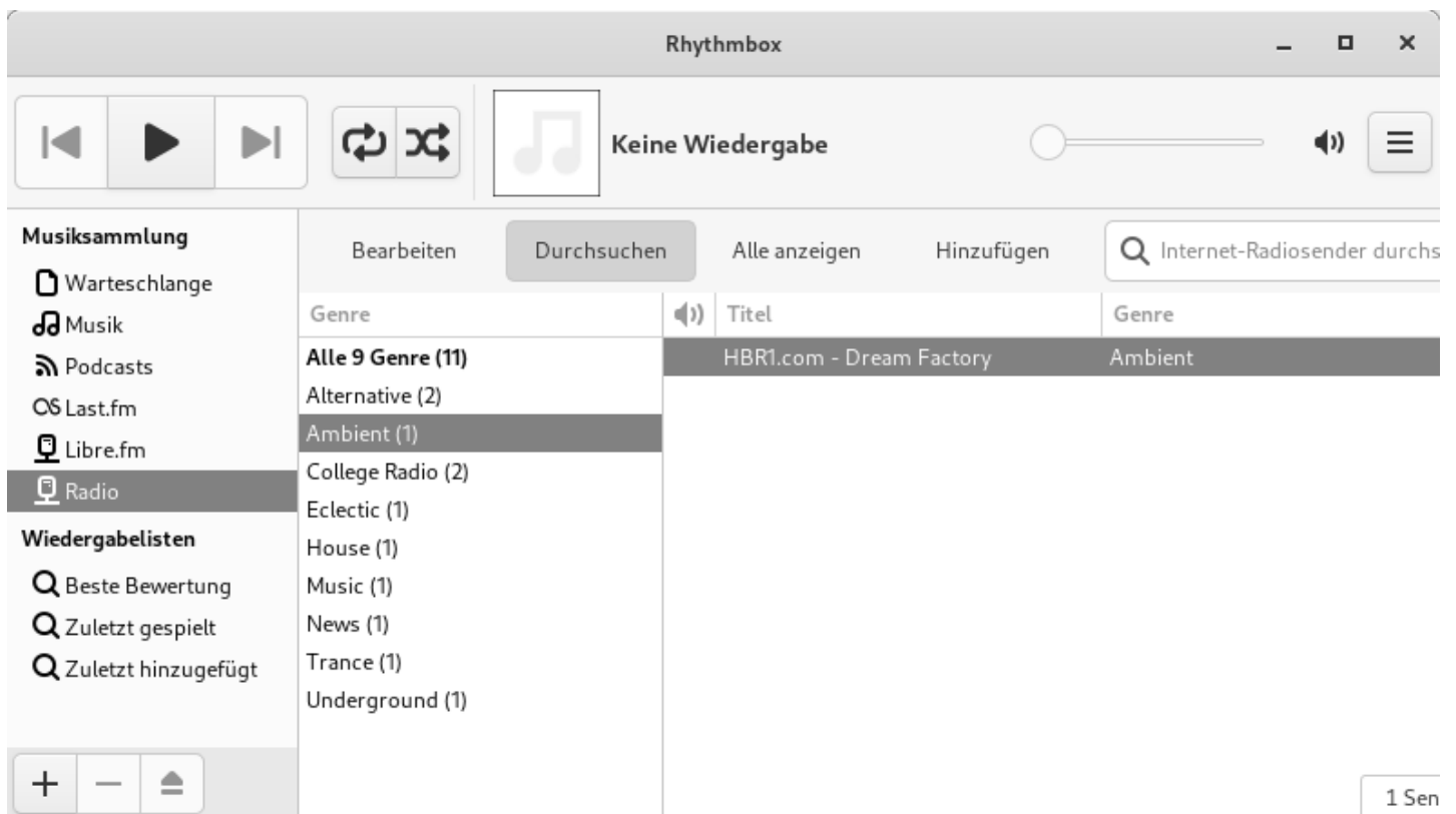
Rhythmbox: Standardansicht
