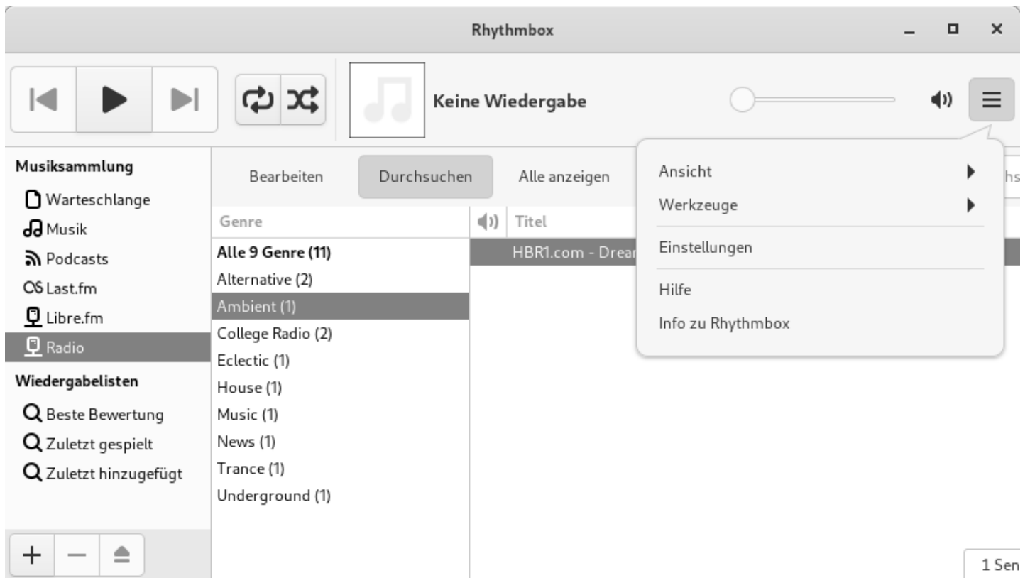
Rhythmbox: Menü
