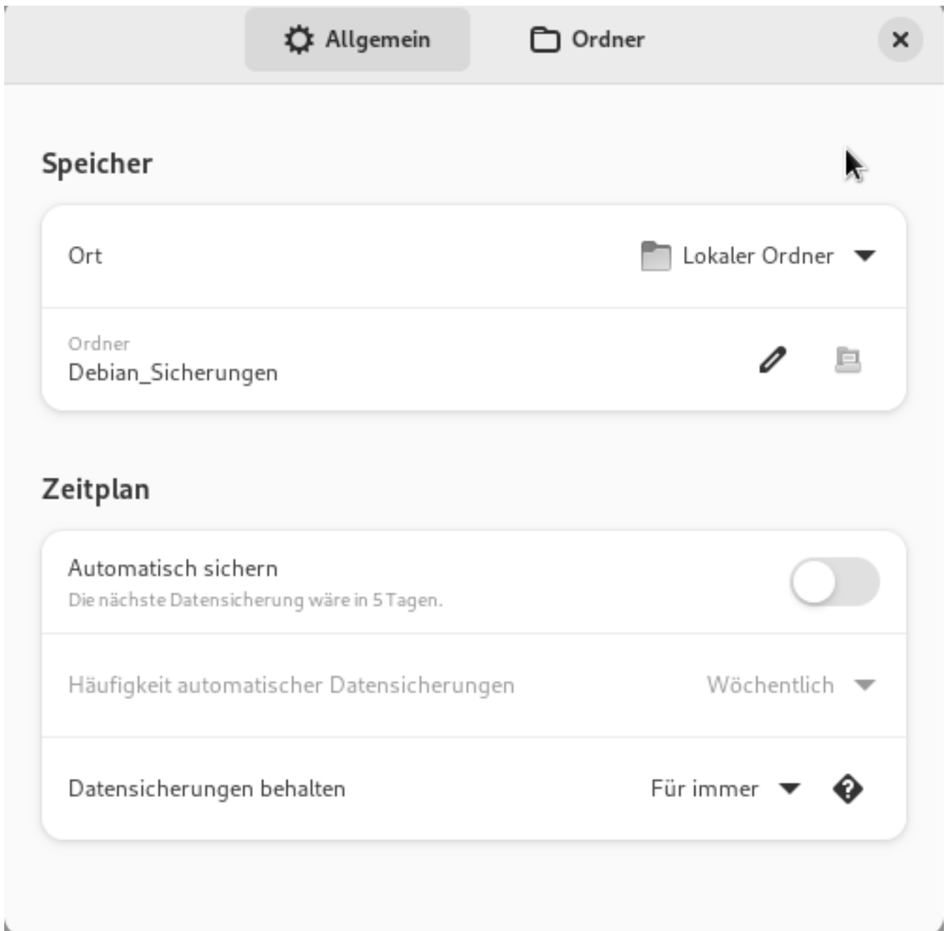
Deja-Dup: Einstellungen
