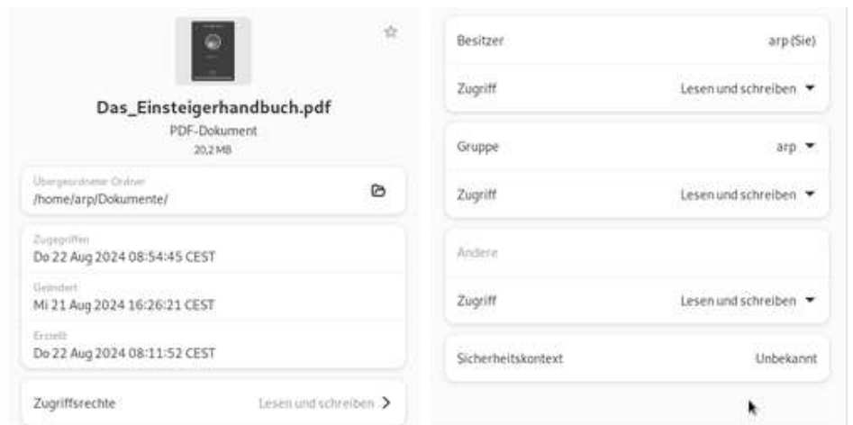
Kontextmenü: Eigenschaften
