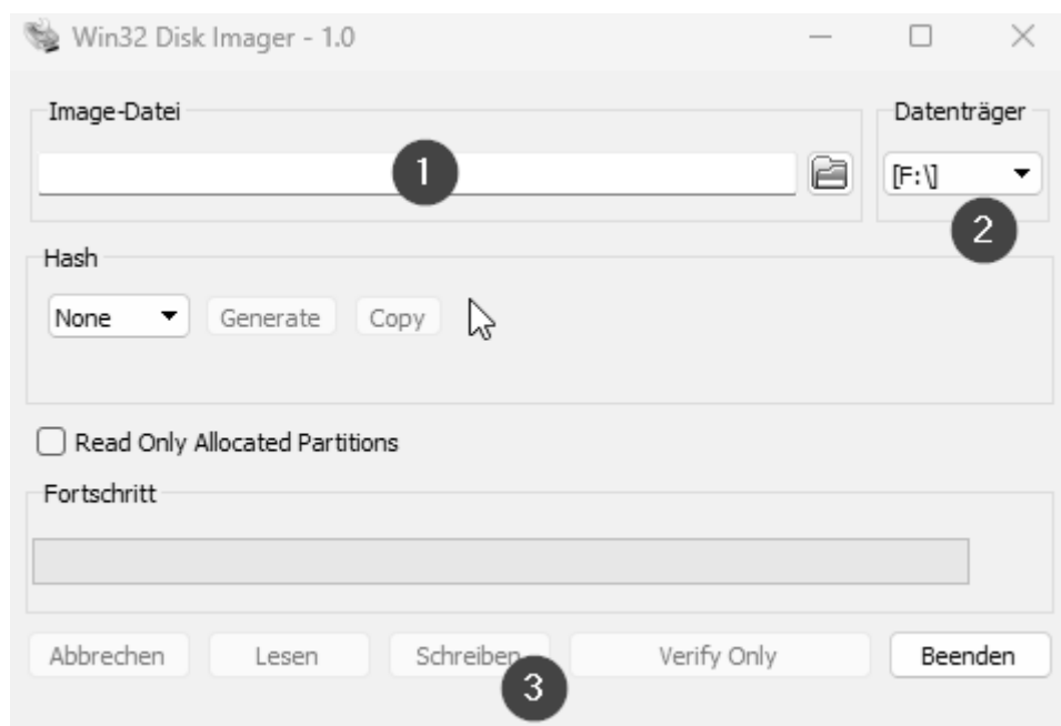
Win32DiskImager
