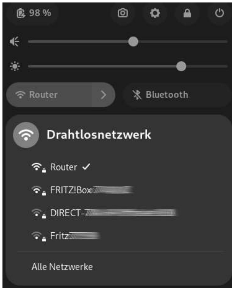
Netzwerkauswahl
