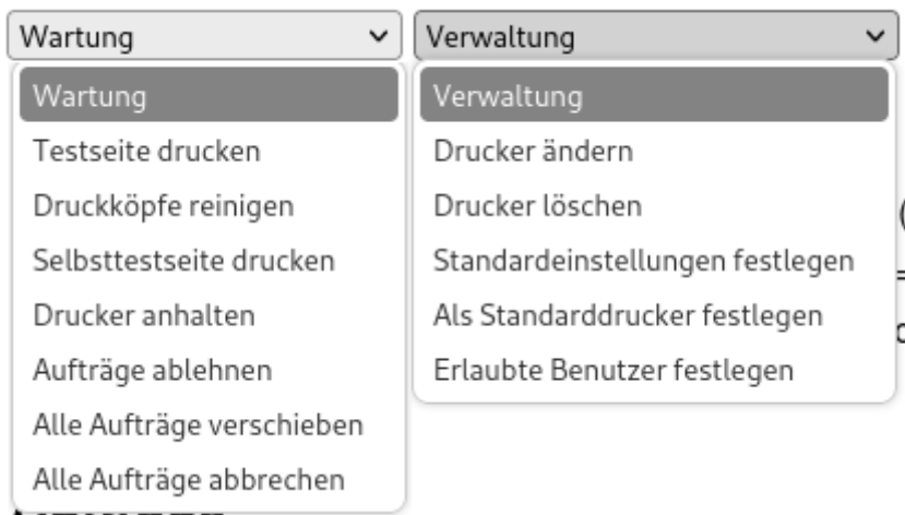
CUPS - Druckerkonfiguration
