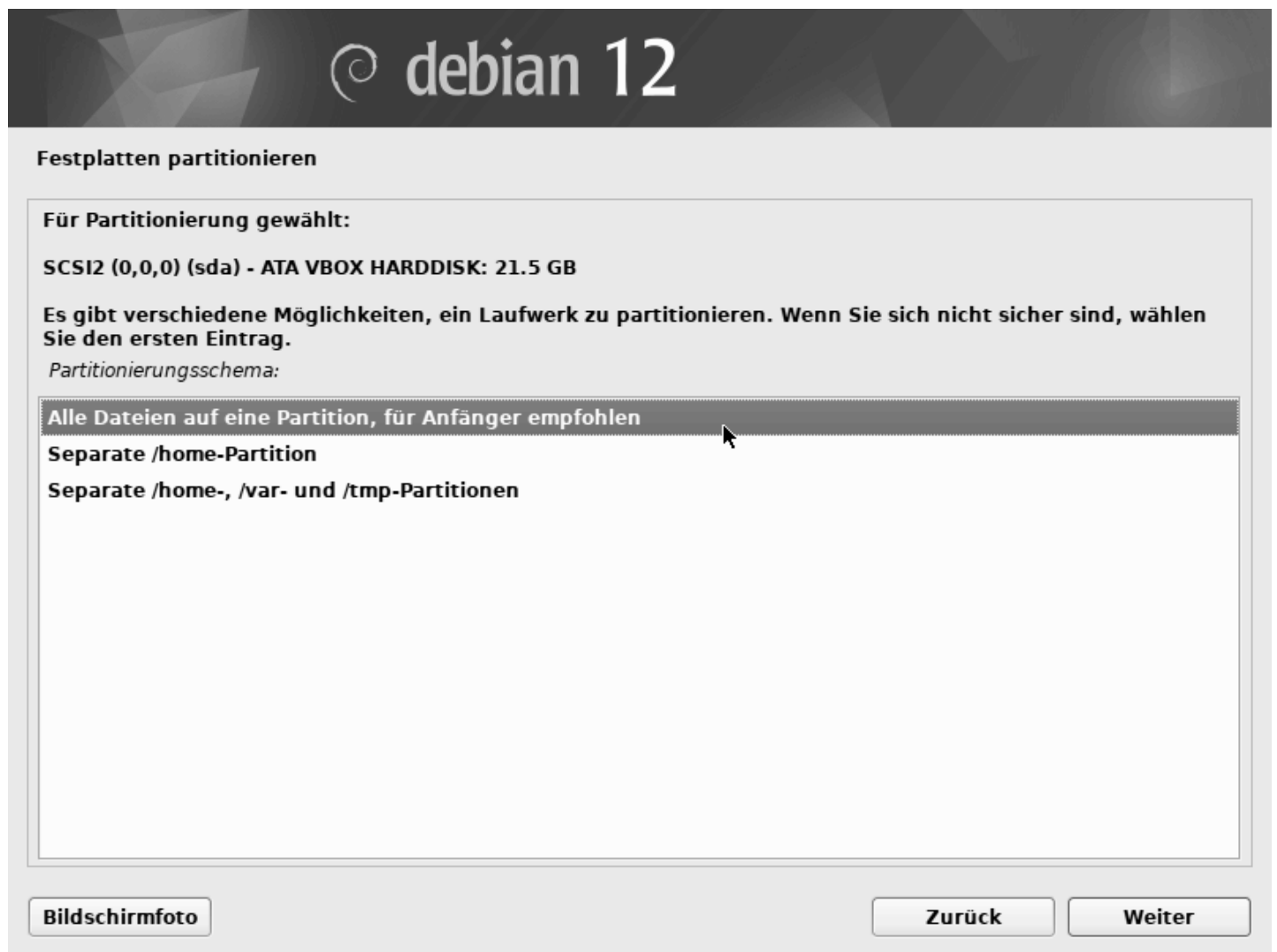
Installation: Partitionierungsmethode
