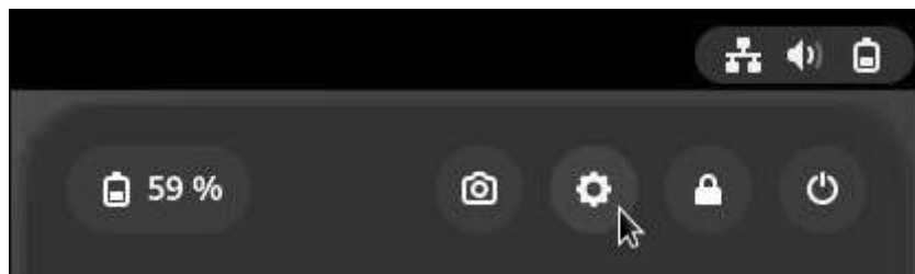
Gnome - Einstellungen
