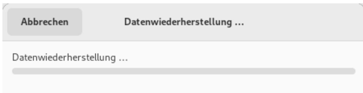
Deja-Dup: Wiederherstellung
