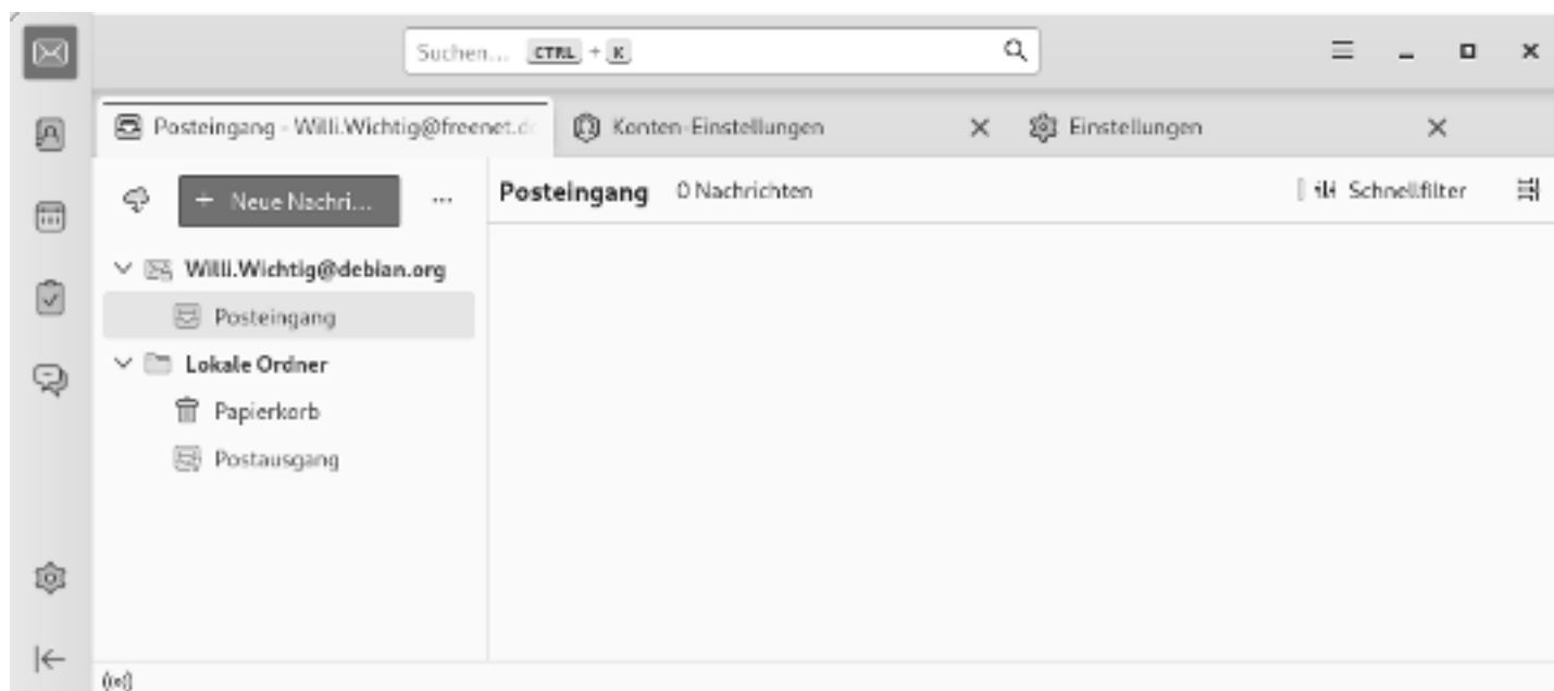
Thunderbird: Standardanzeige
