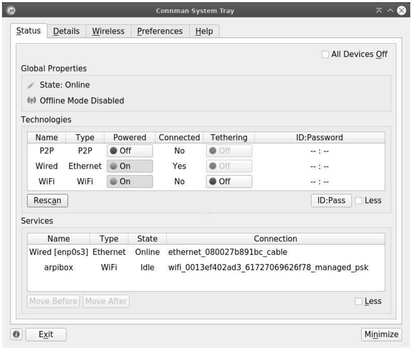
ConnMan: Hauptfenster
