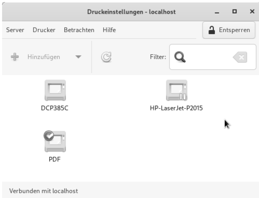
System-config-printer: Standardanzeige
