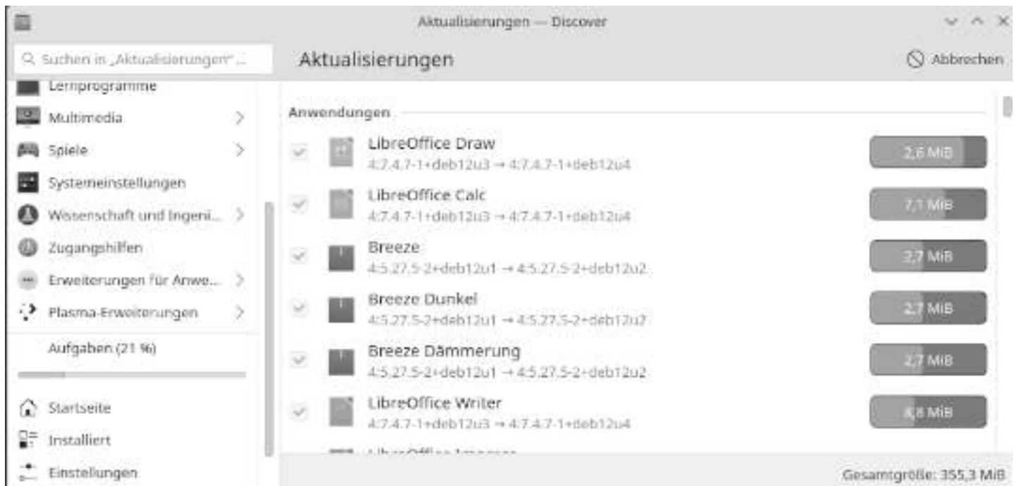
Discover: Aktualisierungsfortschritt
