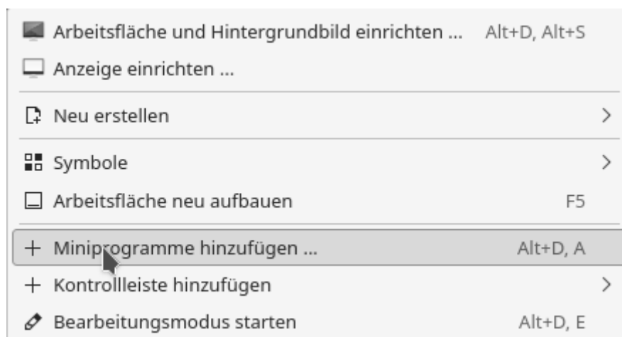
KDE - Widgets
