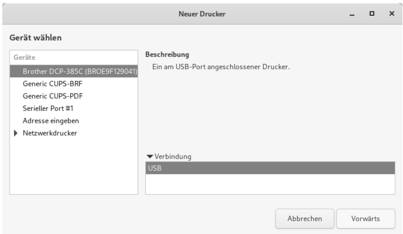
Druckerauswahl
