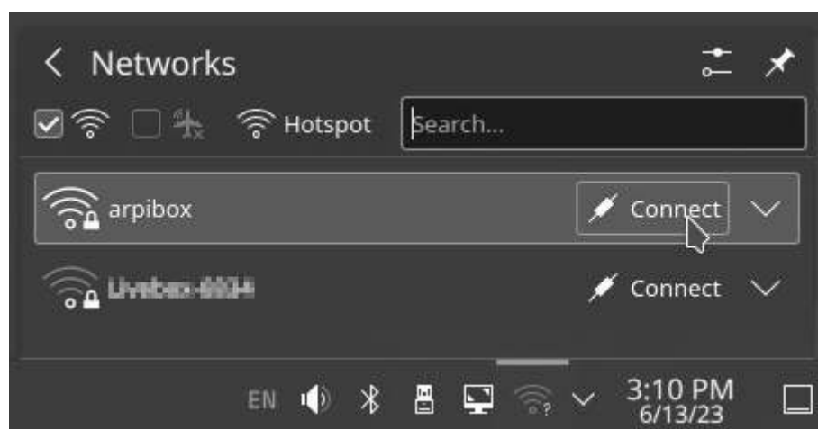
KDE: Netzwerkauswahl
