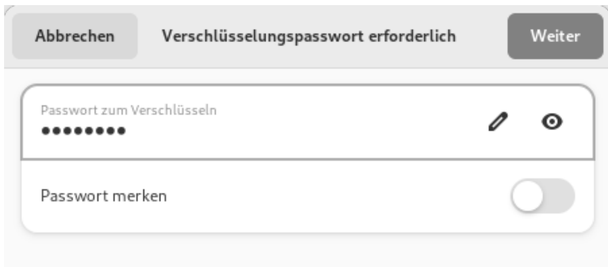
Deja-Dup: Passwortabfrage
